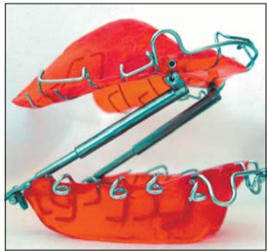
So sieht die neuartige Spange aus. Auffällig sind die beiden teleskopierenden Federstege aus Titan.
